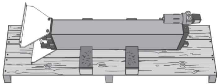
Trockner auf Transportpalette KA-MT6-8
