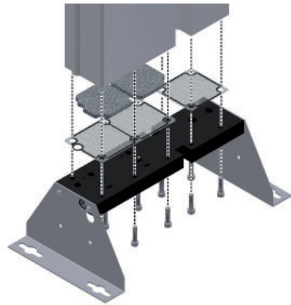
Magnetventilplatte lösen
